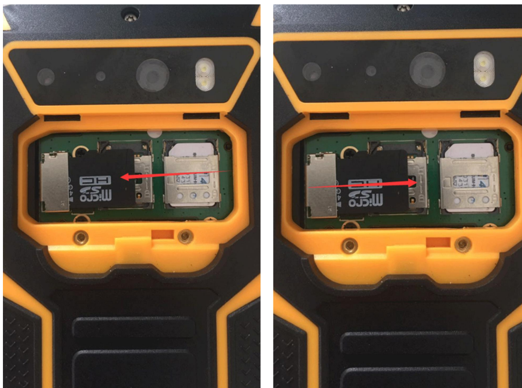
图 2.5-1 移除 T-flash 卡示意图
